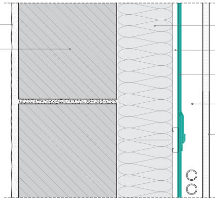
Coupe verticale
