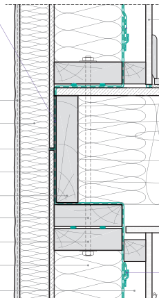
Coupe verticale
