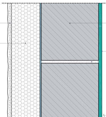
Coupe verticale
